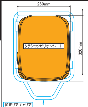
SP武川製クラシックシート SP武川製パッセンジャー用バックレストキット SP武川製サイドバッグサポート同時装着
