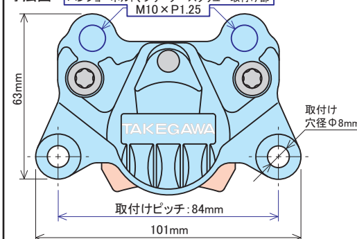
寸法図 バンジョーボルト、ブリーダースクリュー取付け部 M10×P1.25
