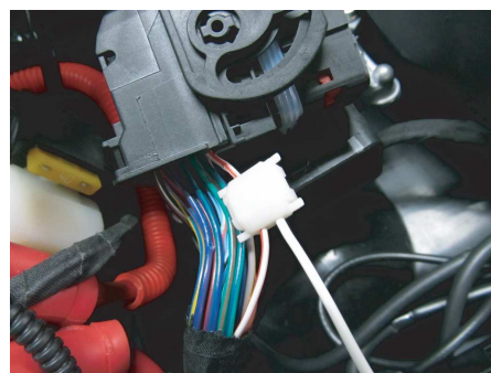
配線の接続先は、シート下のECUカプラーハーネス。
