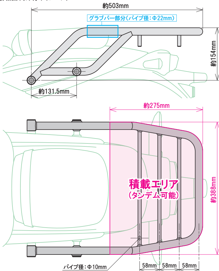
詳細図(取り付けイメージ)
