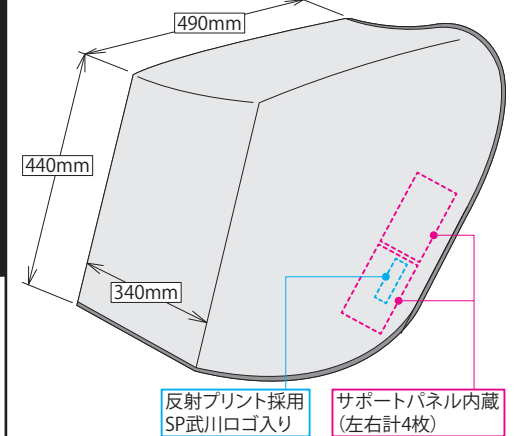
詳細図
