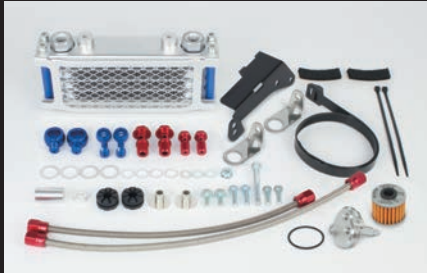
4フィン5オイルライン (07-07-0436)
