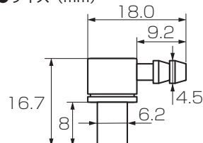
マニホルドのオイル / 負圧ニップルとして便利な L 型ニップルです。
