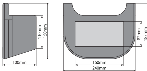
参考寸法図
