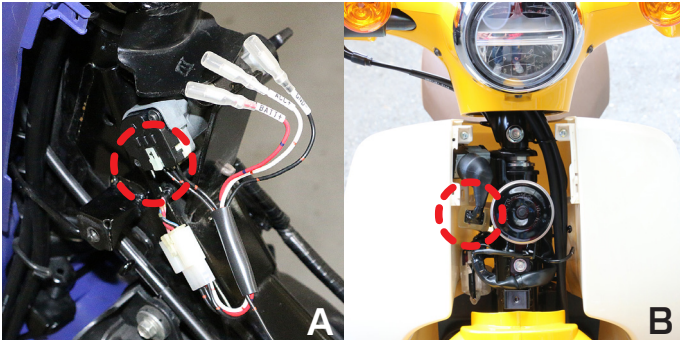
キーシリンダーの 3P カブラーに割り込ませるだけ
