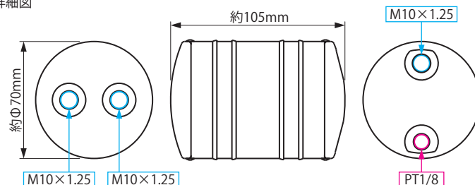
詳細図
