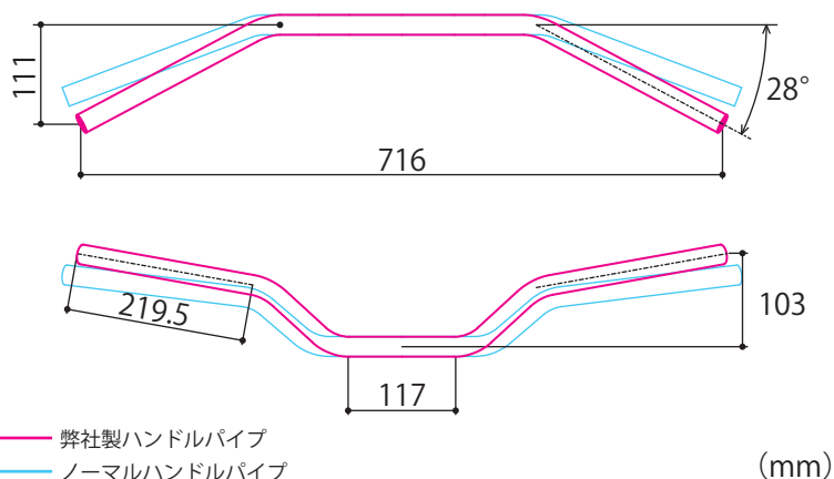
寸法図(ノーマルハンドルとの比較)
